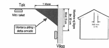
FIGUR 3i – Placering av brandvarnaren
